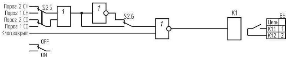
Рисунок 10 – Логика работы реле.
