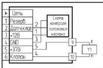
Рисунок 5 – Клапан КЗЭУГ. Схема электрическая принципиальная.
