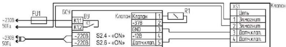
а) схема подключения клапана типа КПЭЭ
