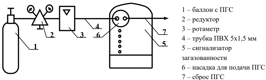
Рисунок Е.1 – Схема для настройки порогов срабатывания
