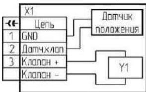
Рисунок 7 – Клапан КЗГЭМ-У.
